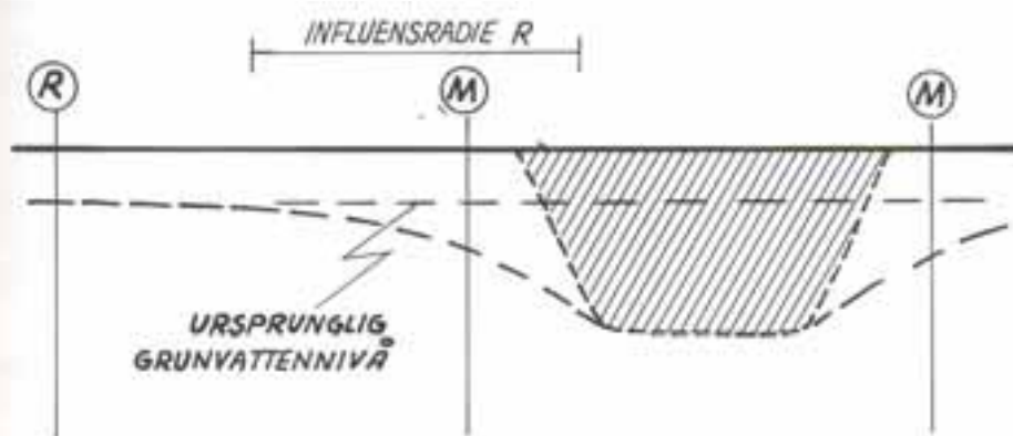
b) vid schaktning med grundvattensänkning
