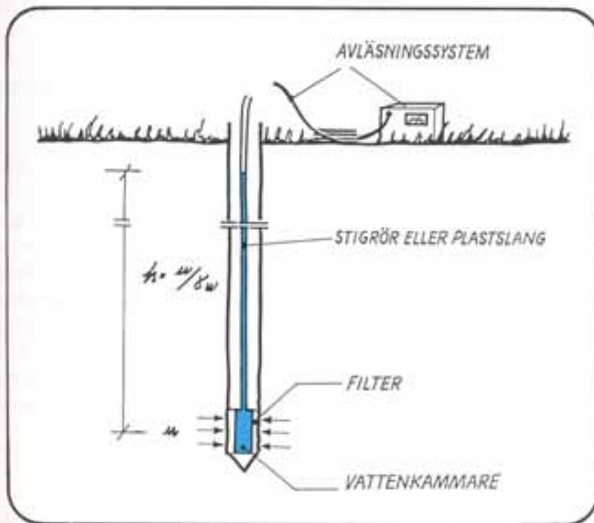
a) öppet system
