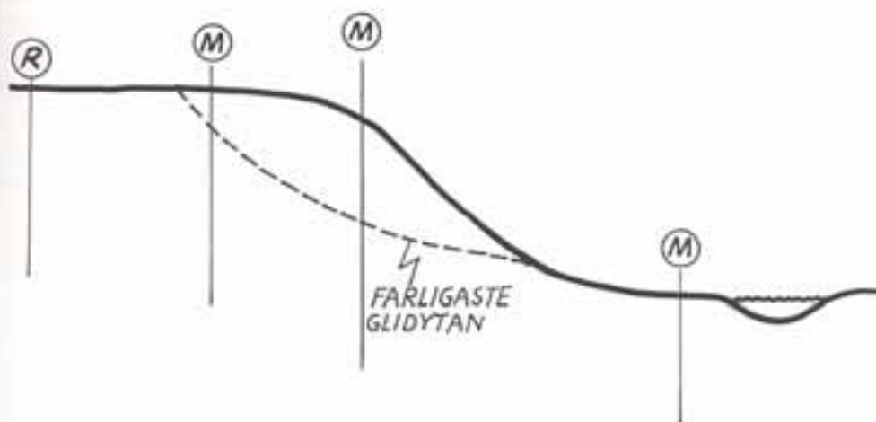
c) vid bevakning av släntstabilitet
