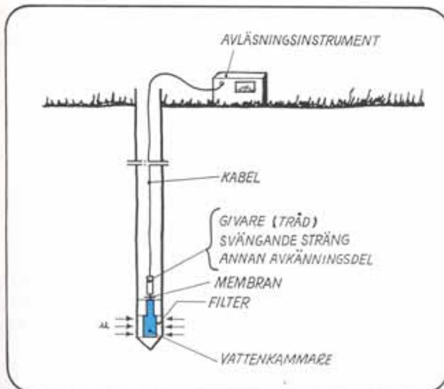
b) slutet system
