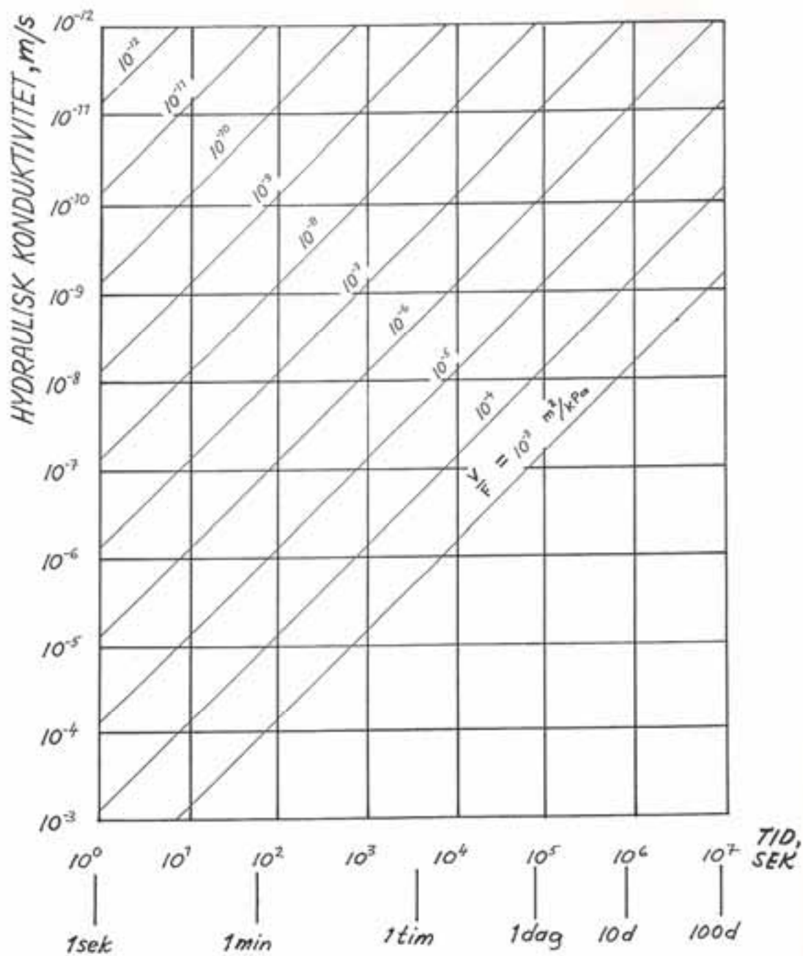
Fig. C4. Diagram för responstid hos olika mätsystem för att uppnå 50% stabilisering (efter CSA, 1971).
